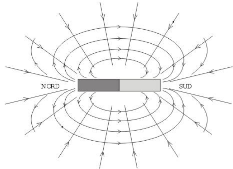
Champ magnétique d'un aimant
