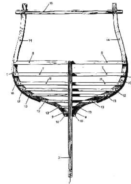
Plan d'une coque de bateau
